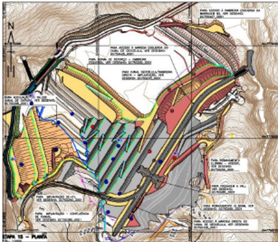
Figura 4 – Arranjo final da descaracterização da barragem B2A, com desmonte parcial da estrutura. (DC750241_0001).
